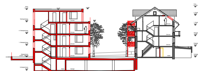
Schnitt A-A
